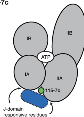
(D) 115-7c and 116-9e control coupling of DnaK_FL to DnaJ
